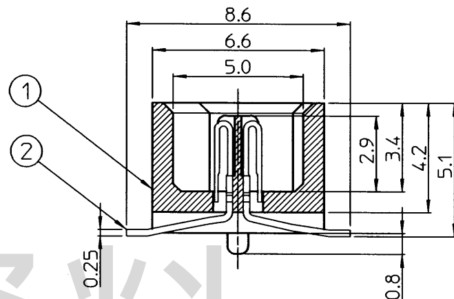
XX' 断面 (尺度 5 : 1)
