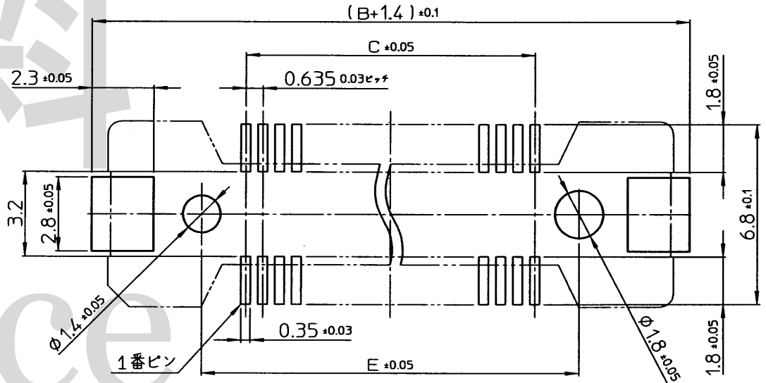
参考基板設計要領(コネクタ搭載面)
